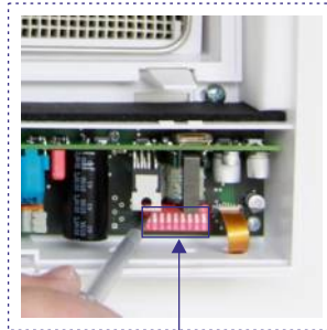
DIP-Schalter
