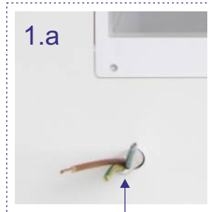
Anschlussleitung NYM-J 3.15
