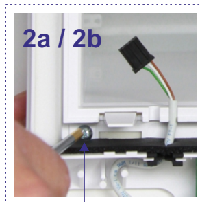
Schrauben 3.9 x 13-16 Design-Gehäuse an der Teleskopeinheit festschrauben
