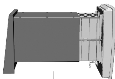
Fassadenabschluss FA-LAW Plus Rohbau-Teleskop-Set TE-LAW Plus Geräteeinheit V-WRG Plus
